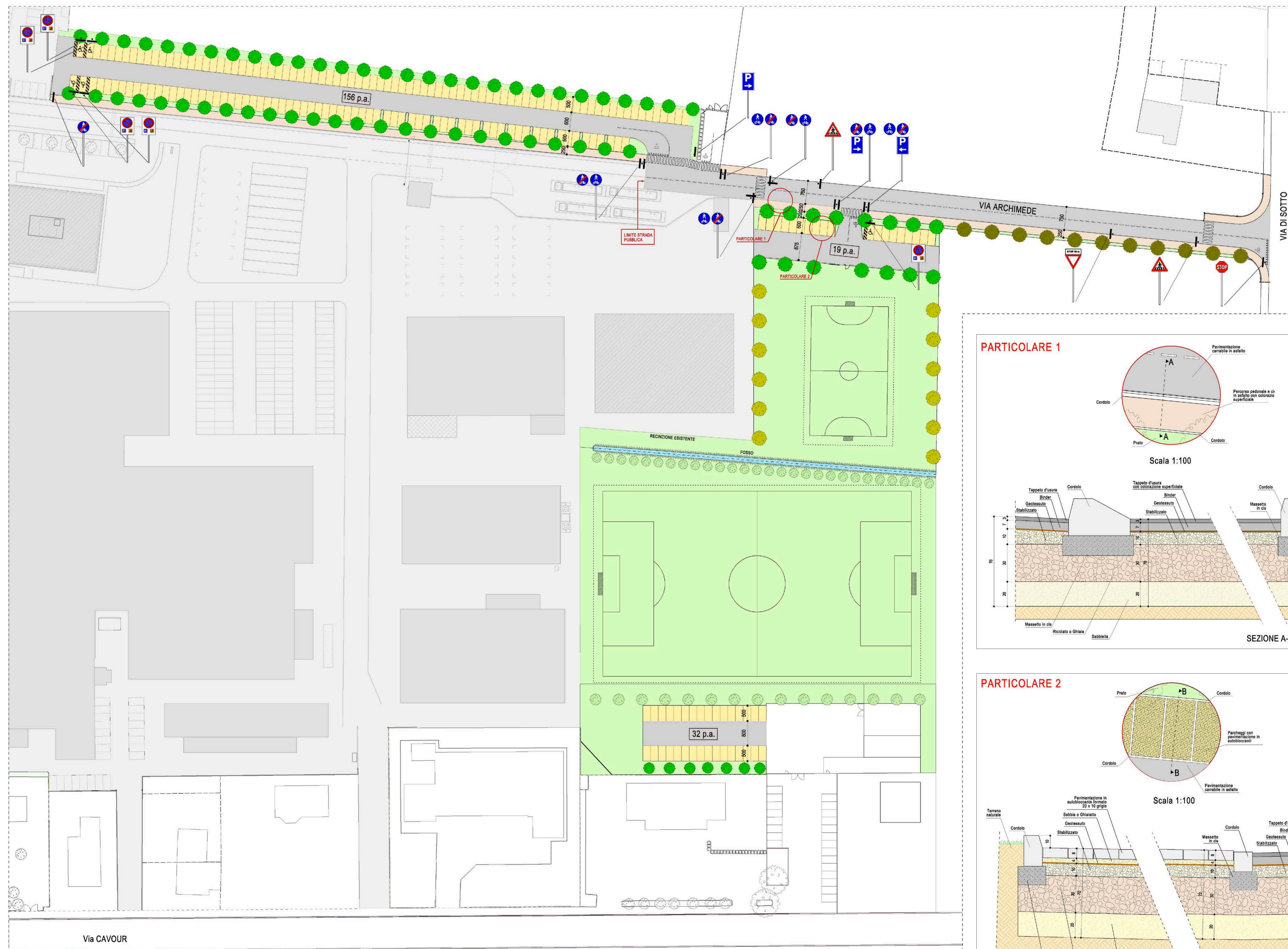
PROGETTO DELLA STRADA E DEL PARCHEGGIO PUBBLICO Scala 1:400
