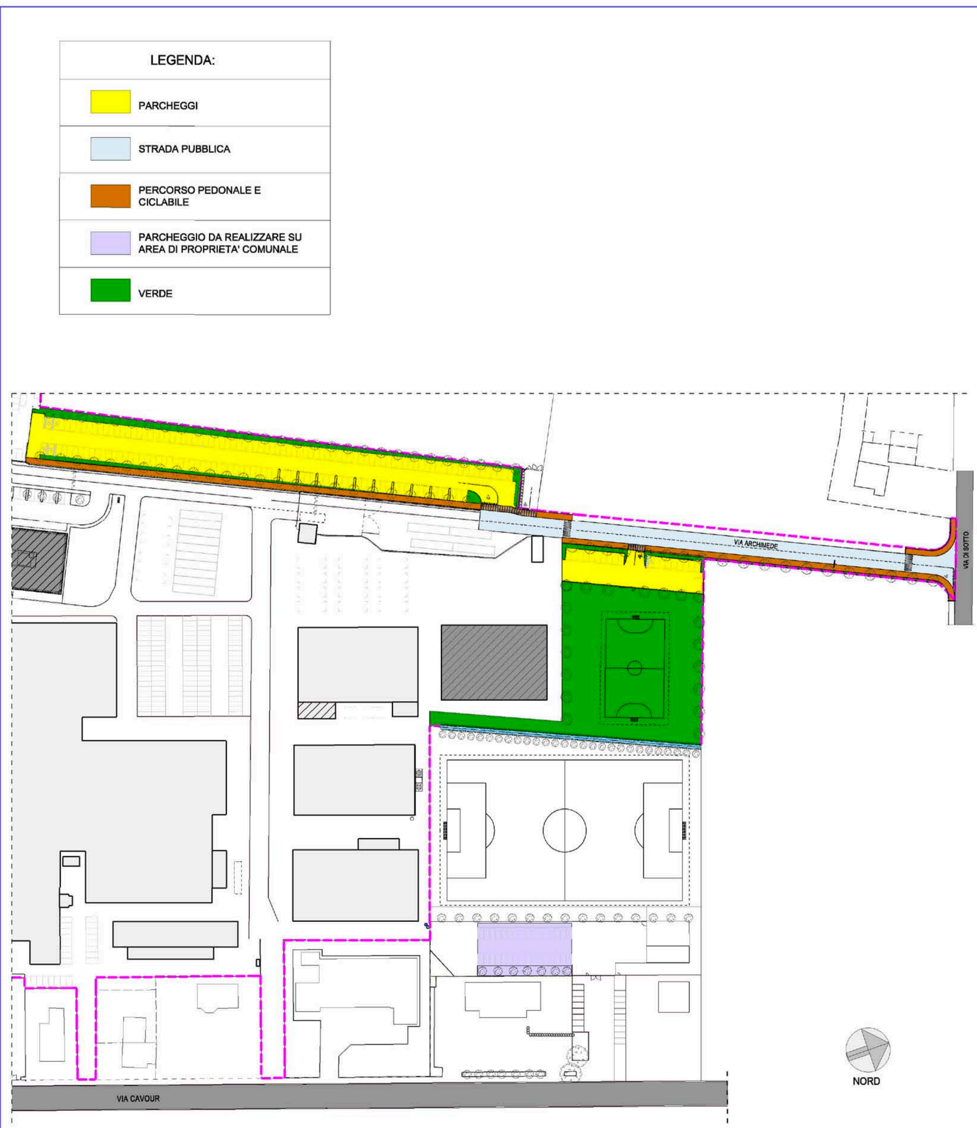
PLANIMETRIA DI INDIVIDUAZIONE DELLE AREE DI PROGETTO Scala 1:1000
